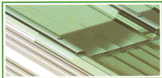
PARTICOLARE DI FISSAGGIO E SORMONTO IN FALDA
