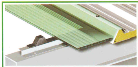
PARTICOLARE DI FISSAGGIO E SORMONTO SU PANNELLO METALLICO
